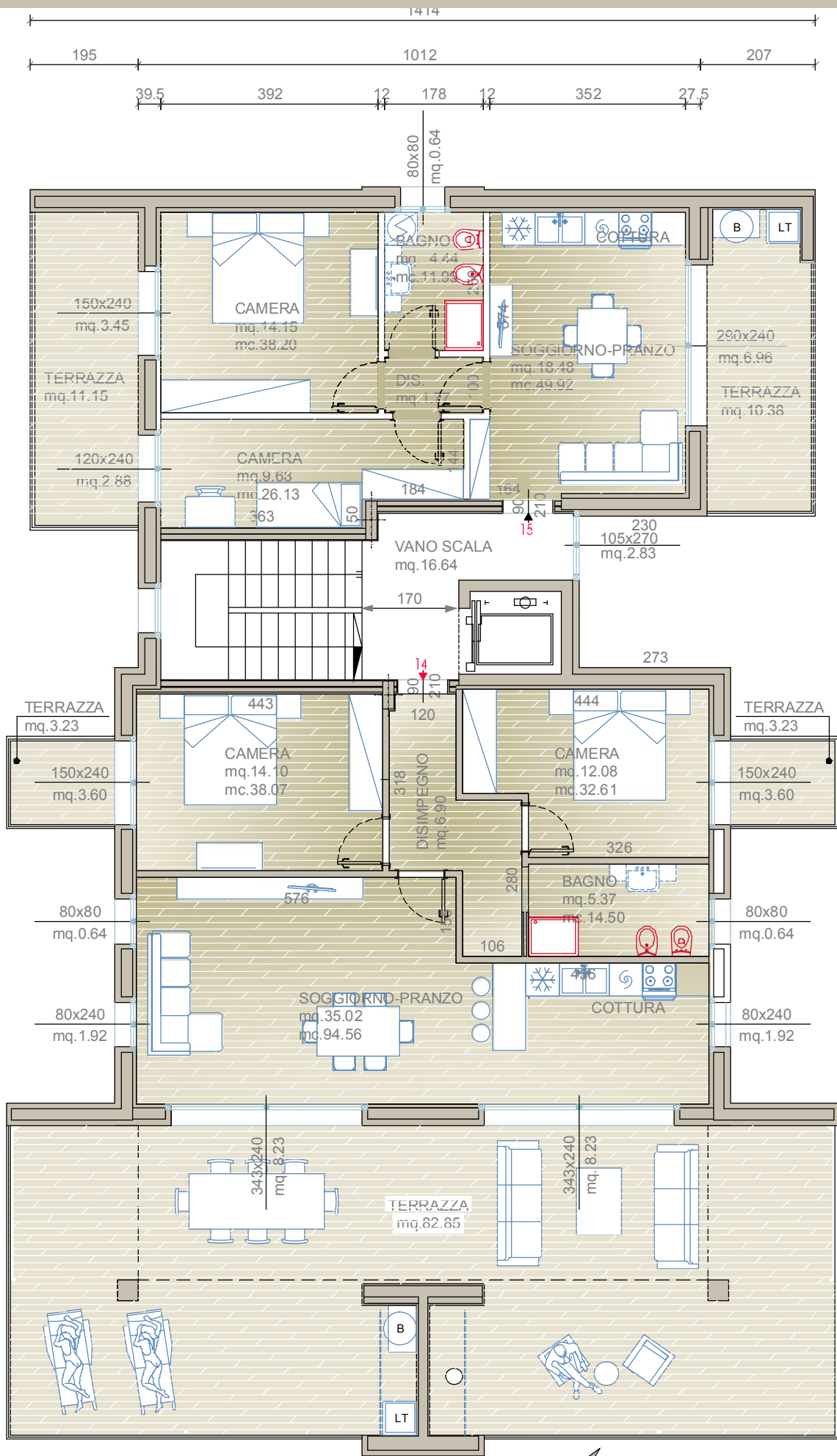
PIANTA PIANO V°
